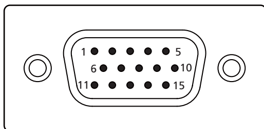
15 ピンカラーディスプレイ信号ケーブル
