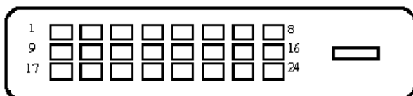
Cavo segnale schermo a colori a 24 pin
