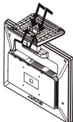
Rysunek 1 Instalacja i demontaż podstawki obrotowej Wspornik(Tylko AL1917 h/AL1917 r)
