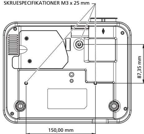
SKRUESPECIFIKATIONER M3 x 25 mm
