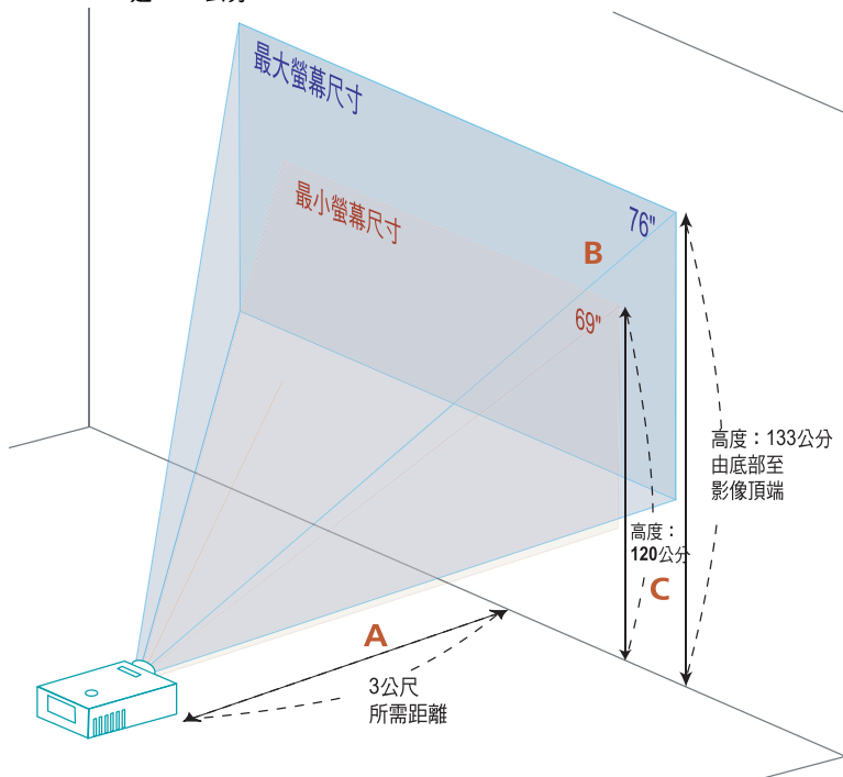
圖：固定距離下，不同的焦距及螢幕尺寸。（僅適用於 X1260 系列，X1160 系列為固定焦距鏡頭）
