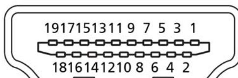
19kolíkový kabel signálu pro barevný monitor*
