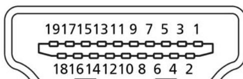
19-bens signalkabel til farveskærm*
