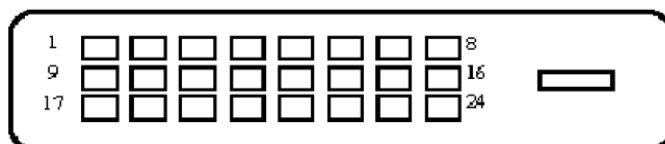
24-bens signalkabel til farveskærm
