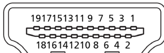
19-nastainen värinäytön signaalikaapeli*
