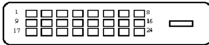
24-nastainen värinäytön signaalikaapeli
