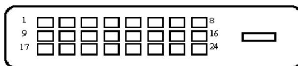
24- pins signaalkabel voor kleurenscherm
