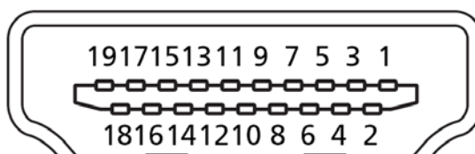
19-pins signaalkabel voor kleurenscherm*
