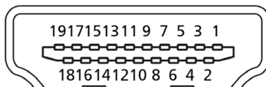
19-pinneres signalkabel for fargeskjerm*
