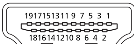
19-Pin Kabel Sygnału Kolorowego Wyświetlacza*
