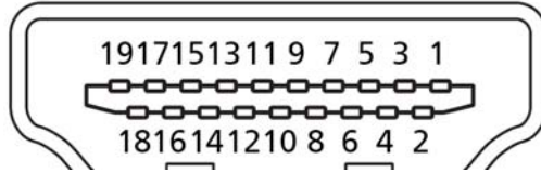
19 pimli renkli ekran sinyal kablosu*
