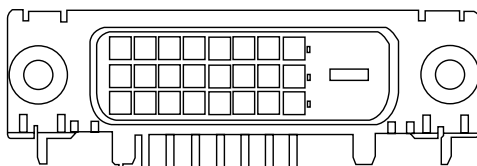
24-pol. Color Display Signalkabel
