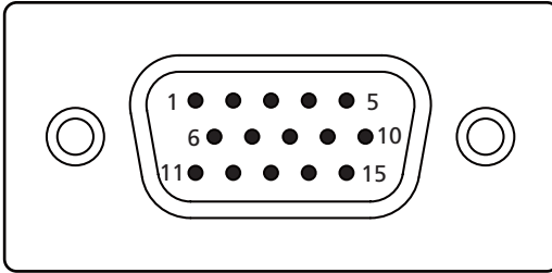
15-pol. Color Display Signalkabel
