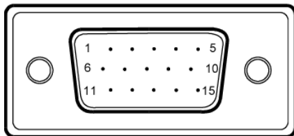
Cable de señal de pantalla en color de 15 contactos
