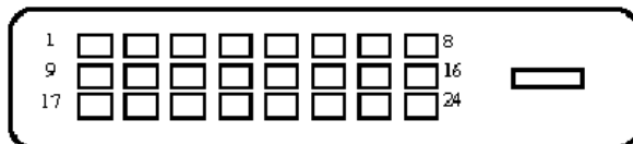
24 kolíkový signálny kábel pre farebné zobrazenie
