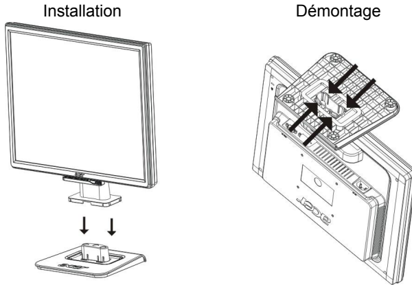
Figure 1 Installation et démontage de la Base Pivotante
