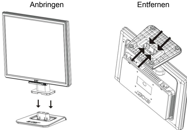
Abb. 1 Anbringen und Entfernen des Fußes
