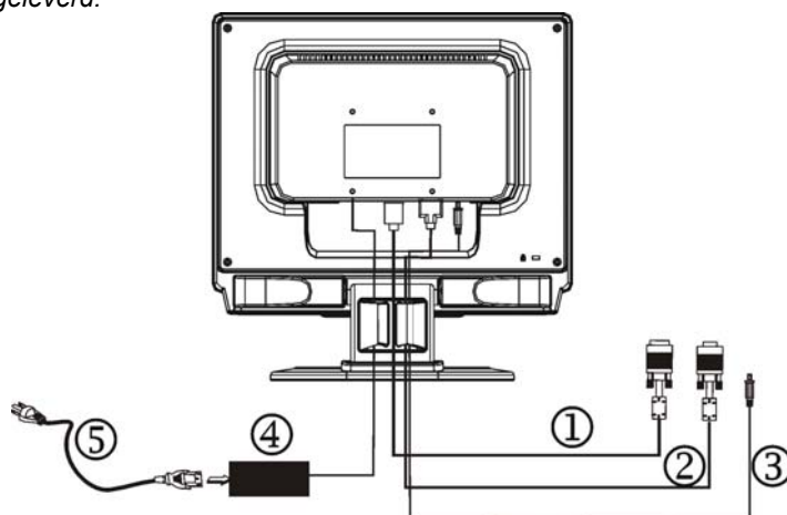
Afbeelding 1 Kabels aansluiten
