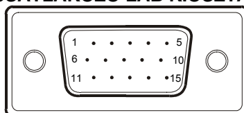
15 - lábú színes kijelző jelkábel
