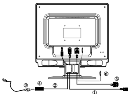
Rysunek 1 Podłączanie przewodów
