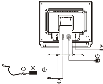
Figura 1 Conexión de los cables
