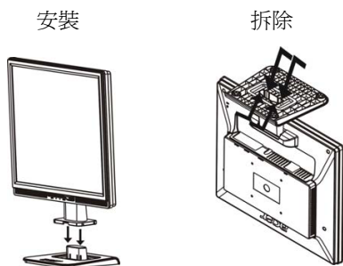
圖一 安裝和拆除轉盤底座
