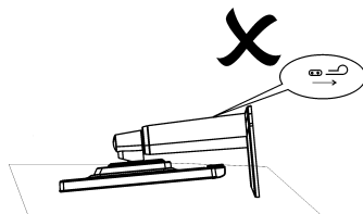
圖一 安裝和拆除轉盤底座
