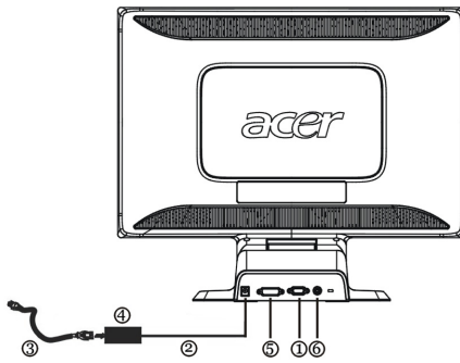
图一 联接线
