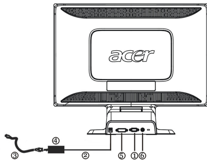
図 1 ケーブルを接続する
