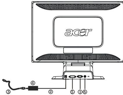
Rysunek 1 Podłączenie przewodów
