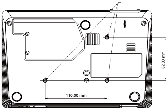
ESPEC. DEL TORNILLO M3 x 20 mm
