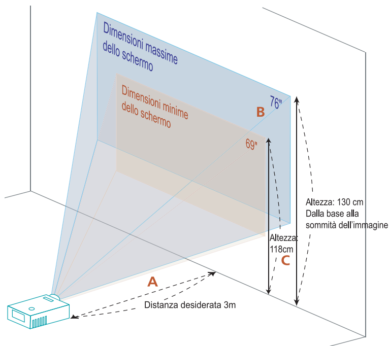
Figura: Distanza fissa con zoom e dimensioni di schermo diverse. (Solo per la serie X1160Z/ZC/PZ/PZC, X1260/Z/ZC/P/PZ/PZC/K/KC, la serie X1160/P ha l'obiettivo fisso)
